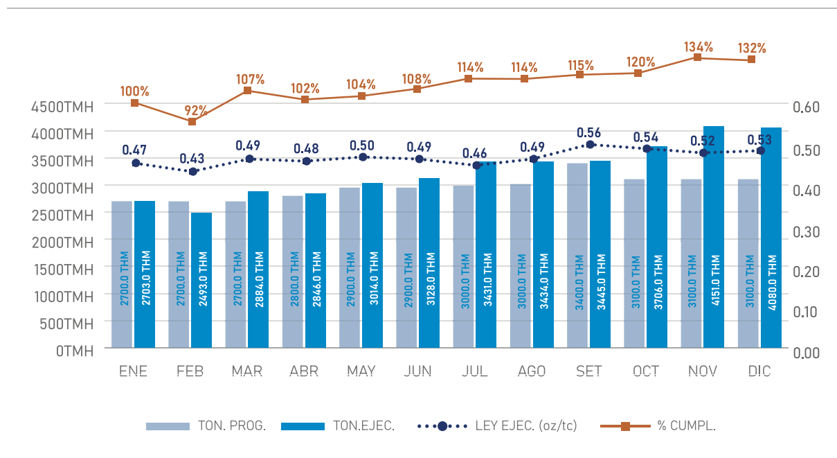
Gráfico N.º14. Tonelaje ejecutado en la Zona 23
