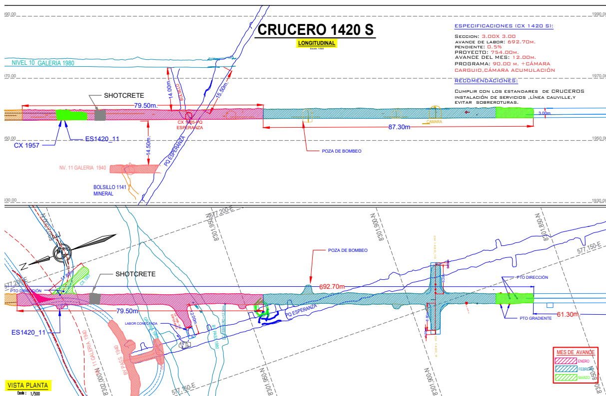
Plano de CX 1420 S actualizado a la fecha 05/01/2024
