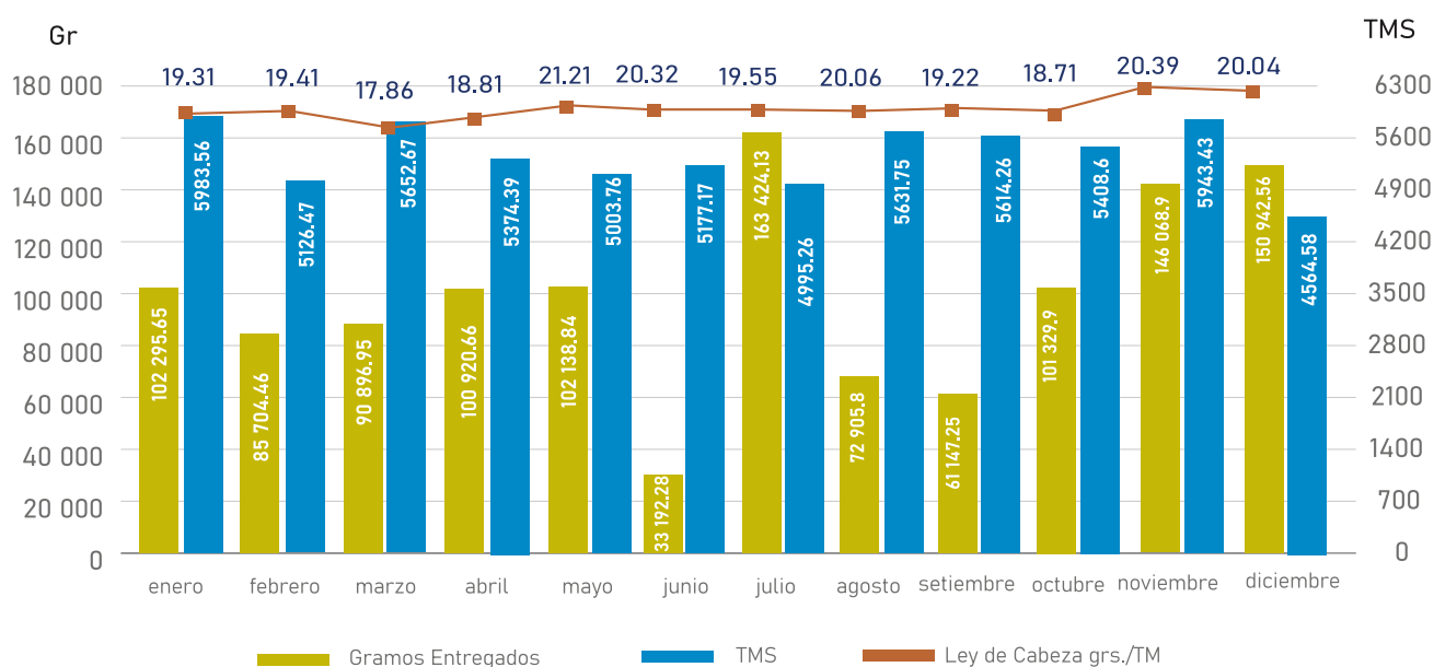
Gráfico n.º 20: Producción Planta de Beneficio Santa Filomena
