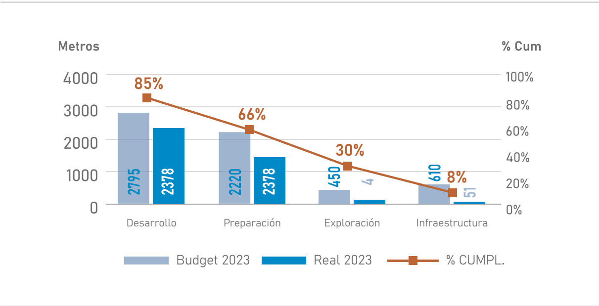
Gráfico N.º8. Avances en metros por fases en Zona 23 y Mina Santa Rosa
