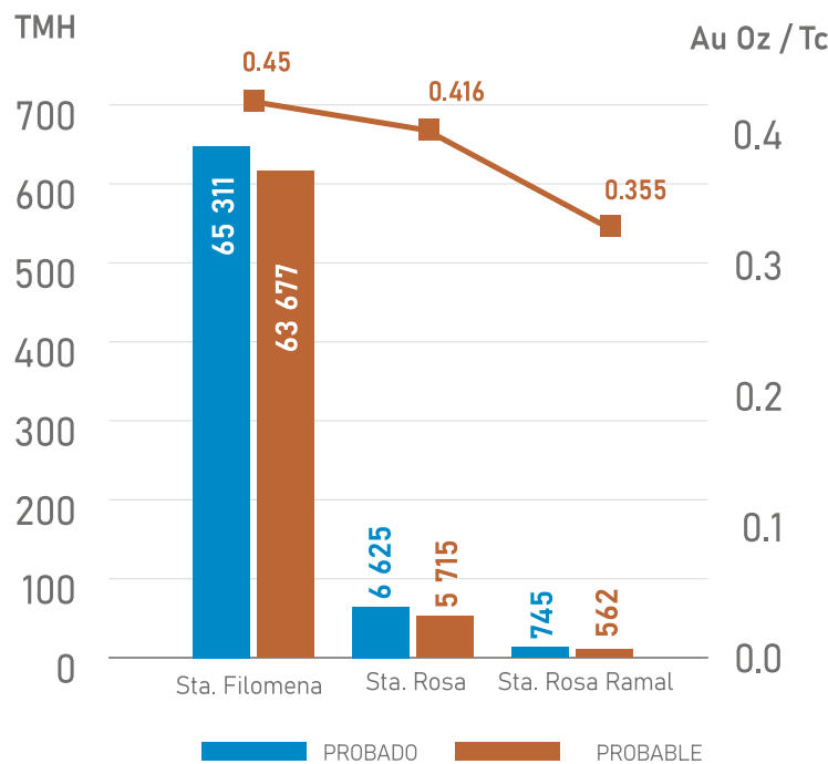
Gráfico n.º18: Reservas de la Mina Santa Filomena (reservas probadas y probables)
